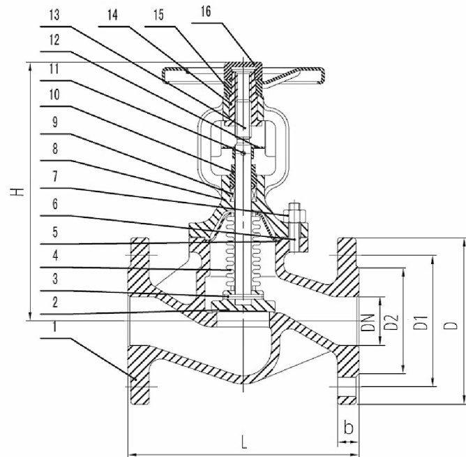
Габаритные и присоединительные размеры, масса
