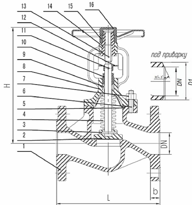
Габаритные и присоединительные размеры, масса
