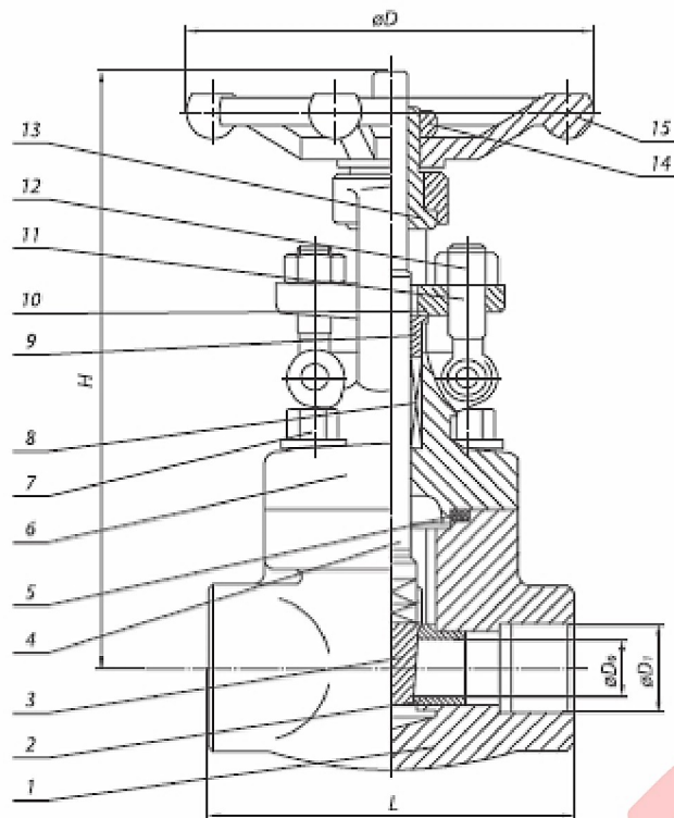
Габаритные и присоединительные размеры, масса
