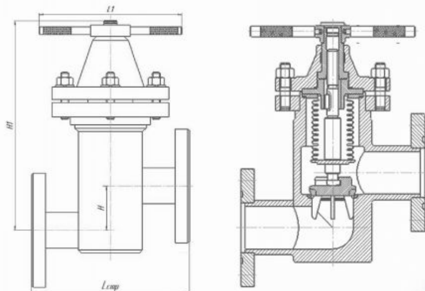
Габаритные и присоединительные размеры, масса
