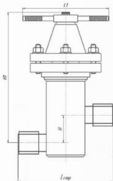
Габаритные и присоединительные размеры, масса
