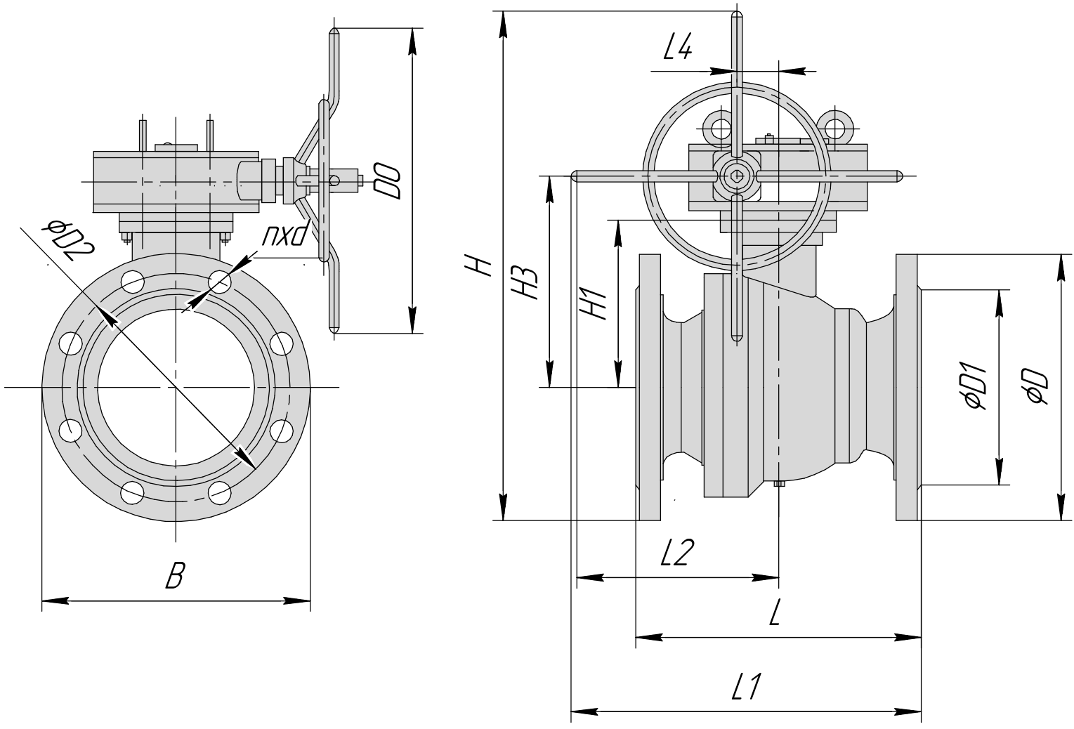
Габаритные и присоединительные размеры, мм:
