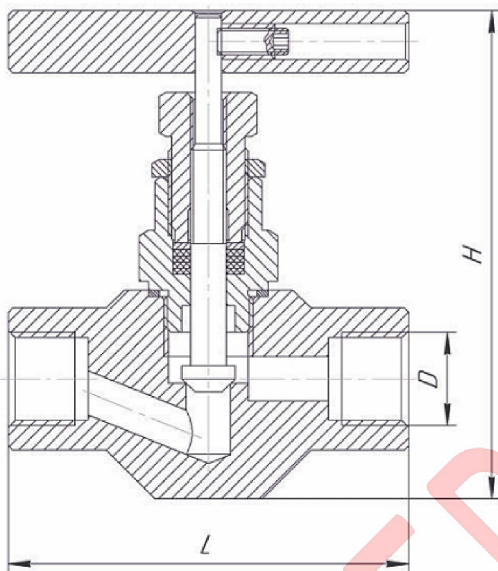
Габаритные и присоединительные размеры, масса
